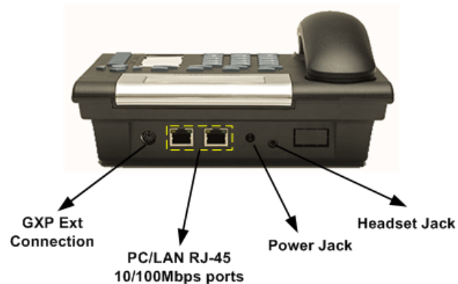
Figura 1: Connettori del GXP2000
